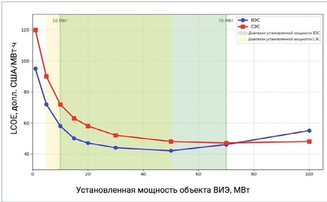
Рис. 2. Зависимость LCOE от установленной мощности ВЭС и СЭС
