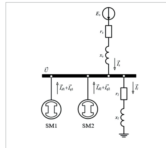
Рис. 1. Эквивалентная схема замещения двухмашинной энергосистемы
