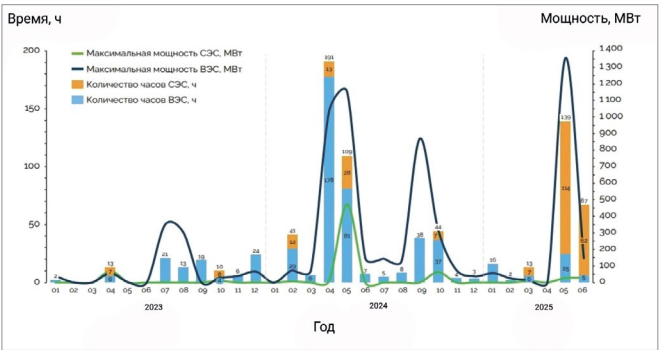
Рис. 5. Длительность и мощность ограничений мощности ВЭС и СЭС в России (2023–2025 гг.)
