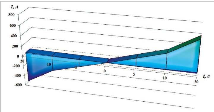
Рис. 2. Пример определения экстремумов функции аварийно допустимой токовой нагрузки ВЛ 110 кВ А — Б при учете реверса токовой нагрузки
