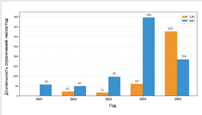
Рис. 4. Динамика ввода ограничений мощности ВЭС и СЭС в ЕЭС России (2021–2025 гг.)
