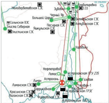
Рис. 6. Принципиальная схема электрических соединений энергосистемы Астраханской области
