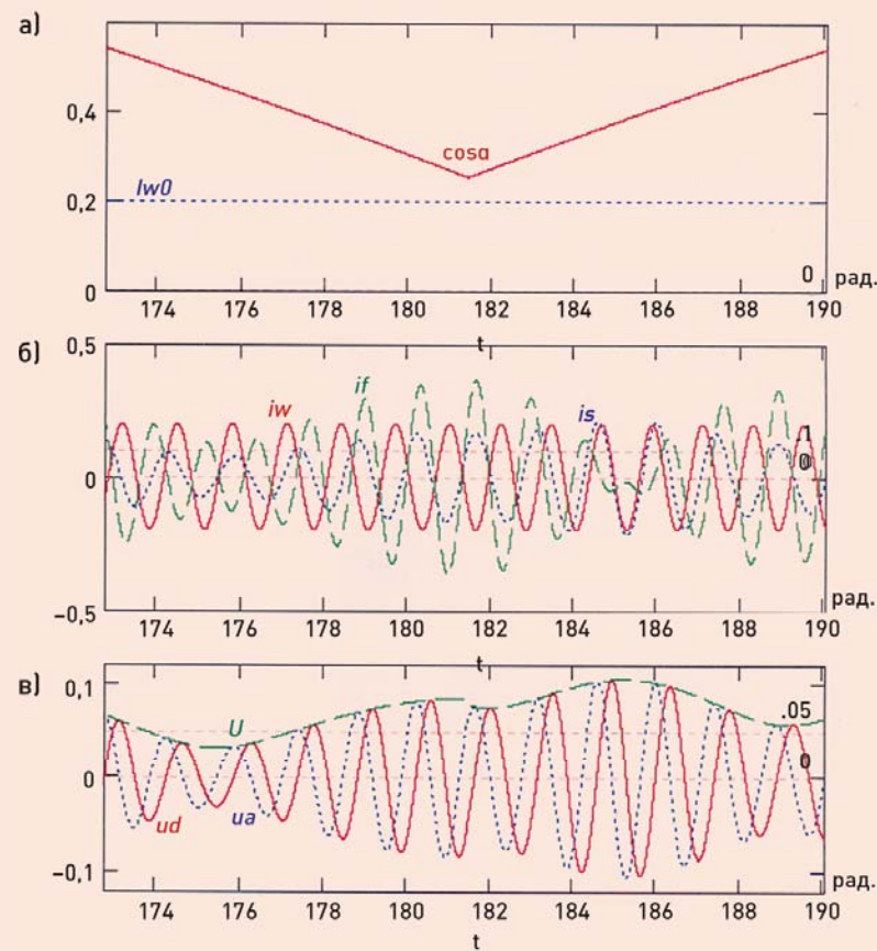
а) амплитуда тока искажений — I_{w0} и косинус угла управления; б) i_s — ток сети; i_w — ток искажений; i_f — ток фильтра; в) U — напряжение на шинах; u_d , u_q — напряжение на шинах в осях d, q
