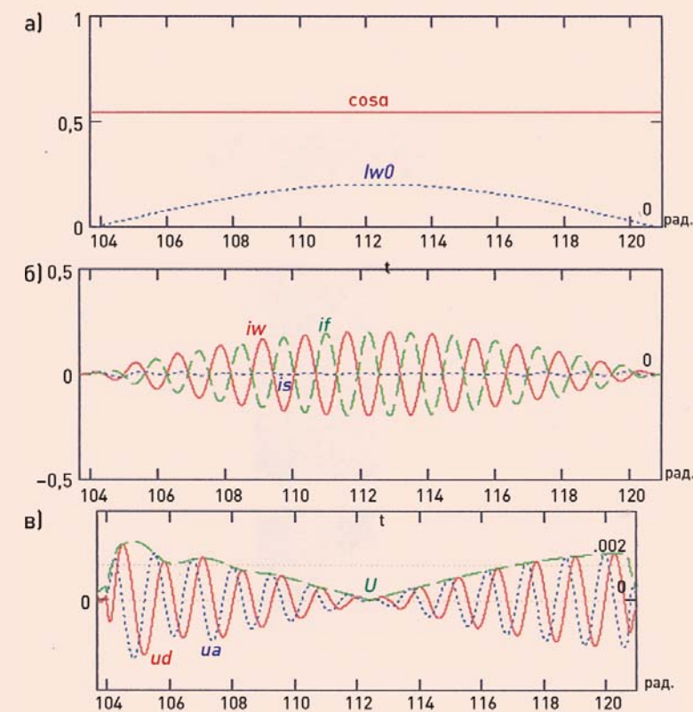
а) амплитуда тока искажений — iw и косинус угла управления; б) is — ток сети; iw — ток искажений; if — ток фильтра; в) U — напряжение на шинах; ud, uq — напряжение на шинах в осях d, q
