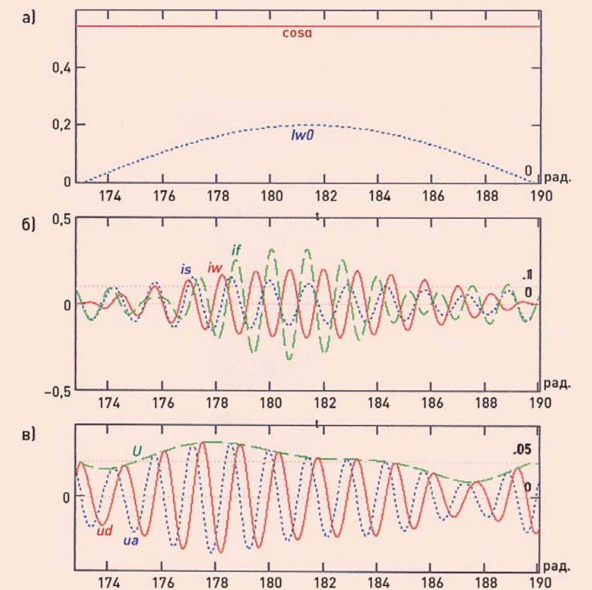
а) амплитуда тока искажений — i_w0 и косинус угла управления; б) i_s — ток сети; i_w — ток искажений; i_f — ток фильтра; в) U — напряжение на шинах; u_d , u_q — напряжение на шинах в осях d , q
